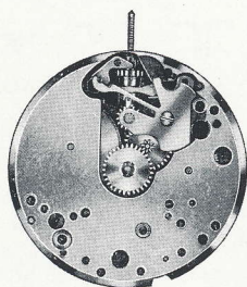
Cal. 6340
